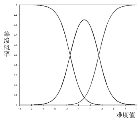
图6 连贯性量表的概率曲线
