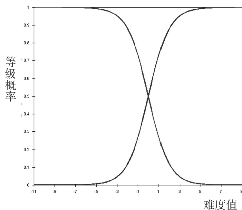
图5 长度量表的概率曲线
