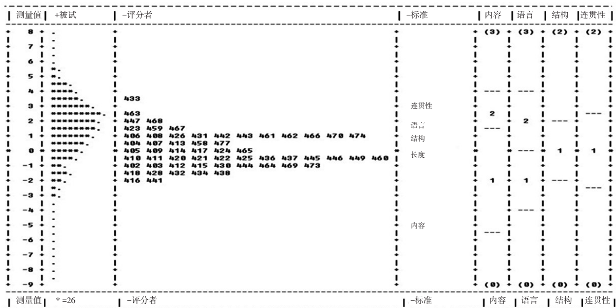
图1 被试参数、评分者参数和评分标准参数的校正图
