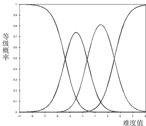
图3 语言量表的概率曲线
