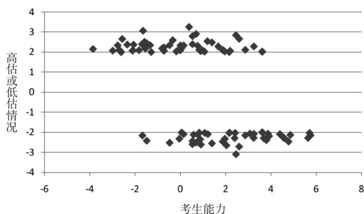
图7 评分者对被试能力的高估或者低估的散点图
