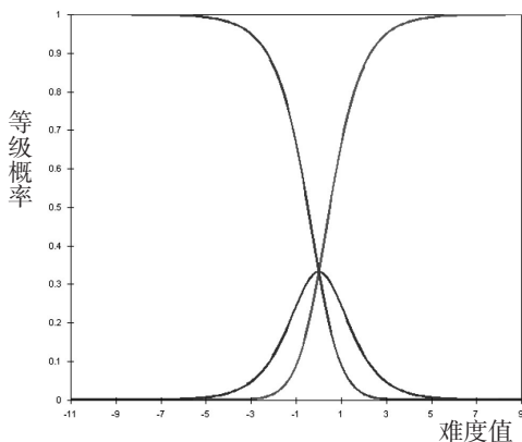
图4 结构量表的概率曲线
