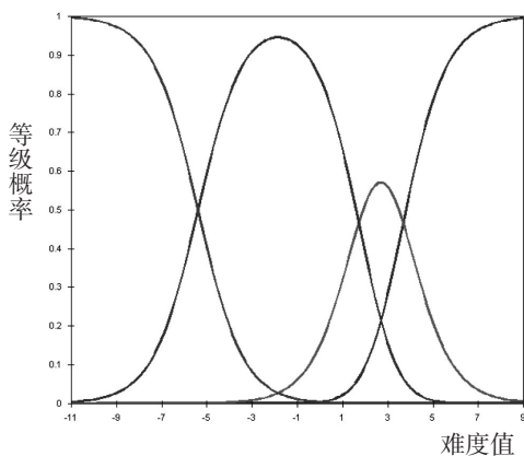
图2 内容量表的概率曲线
